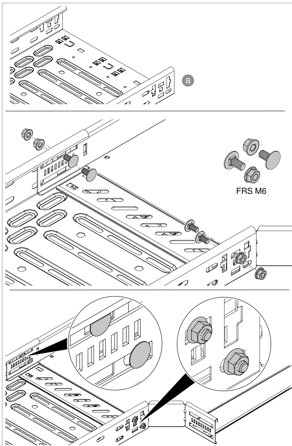
Obr. 48: Upevnění tvarového dílu pomocí šroubů (nedělenému žlabu (a))
