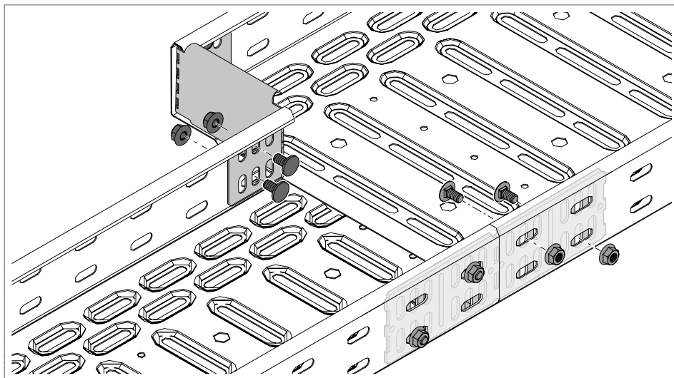
Obr. 74: Montáž podélné a úhlové spojky a redukčního úhelníku
