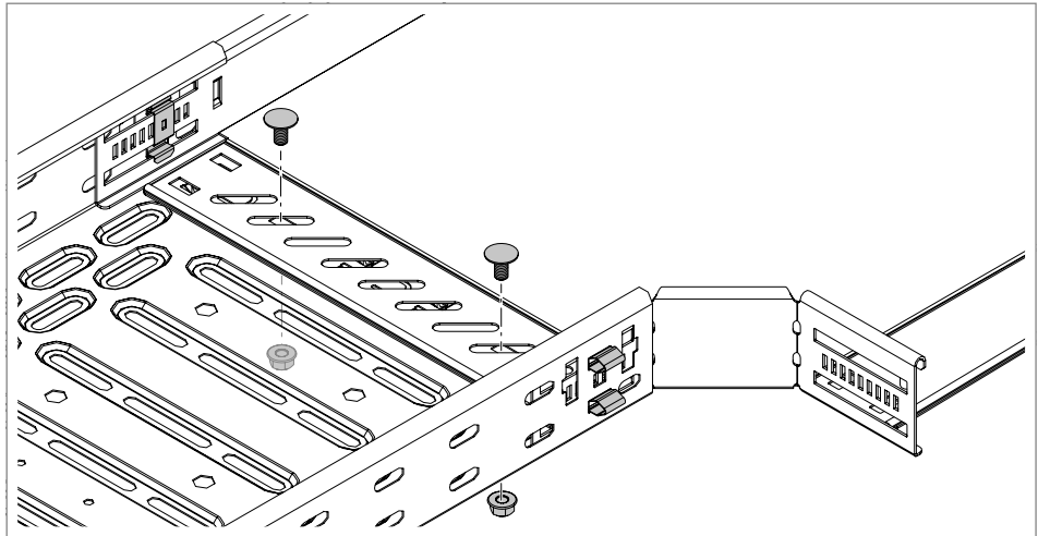
Obr. 47: Přišroubování spojuvací lišty
